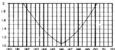
VSWR
